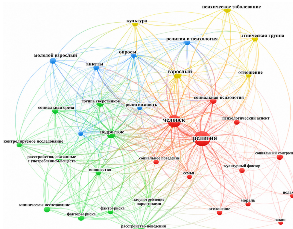
Рисунок 2 Кластерный анализ данных, N=124
